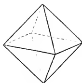
Oктаeder.
